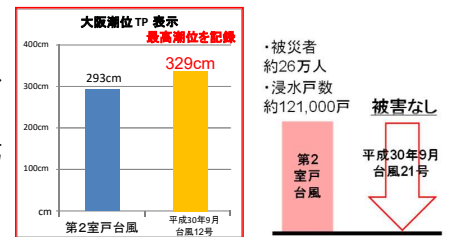
平成30年9月台風21号による毛馬排水機場等の効果
