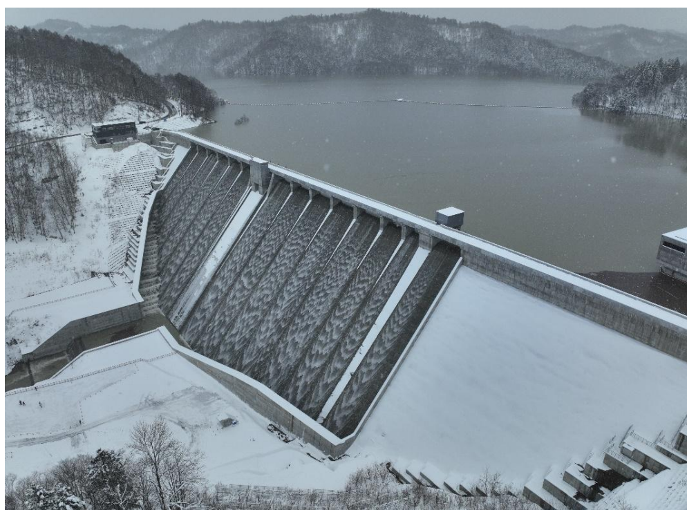
試験湛水が満水に達した新桂沢ダム（令和5年12月）
