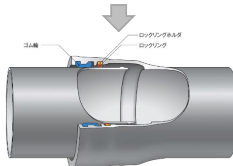
耐震管 (ダクタイル鋳鉄管GX形)
