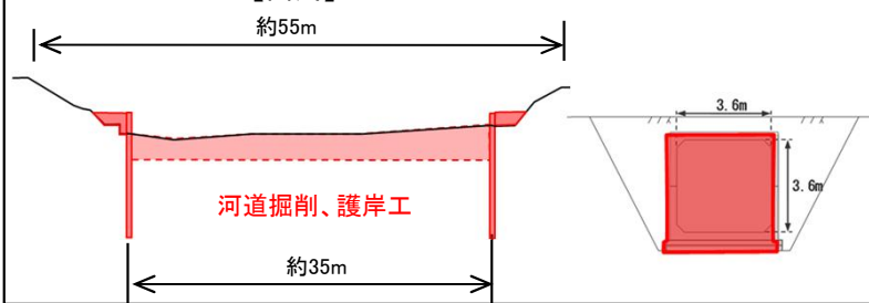
標準横断面図 【西川】 約55m 【下川(放水路)】
